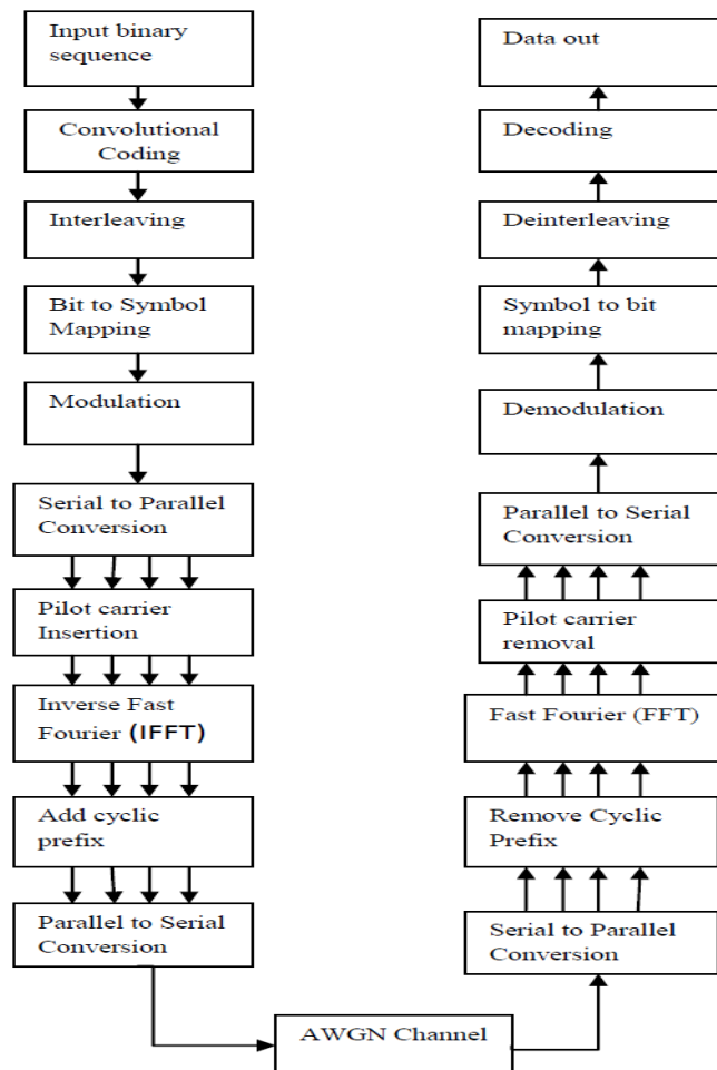
Fig.1 IEEE 802.16 physical layer
